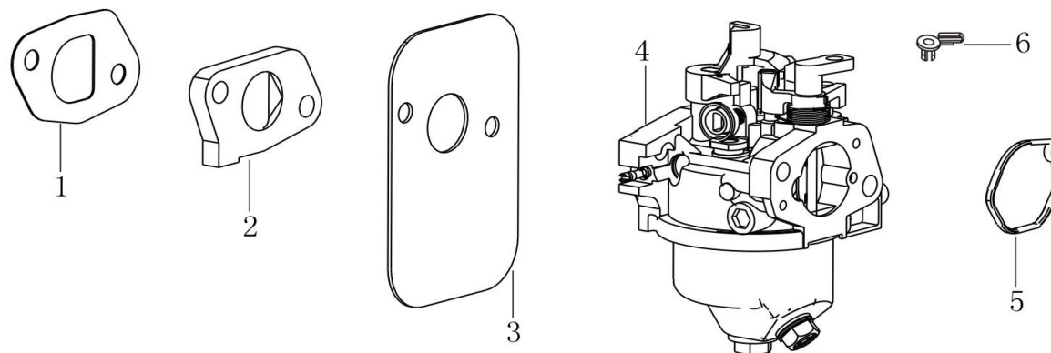
化油器 (CARBURETOR)
